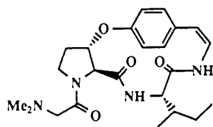
Nummularine F (3)
